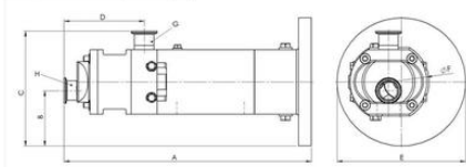
Mått HYGHSPIN Extended kompaktkonstrerad (mm)
