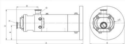
Mått HYGHSPN Extended kompaktsmonterad (mm)
