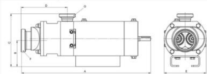
Mått HYGHSPN Extended fl axel (mm)
