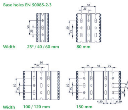
Base holes EN 50085-2-3
